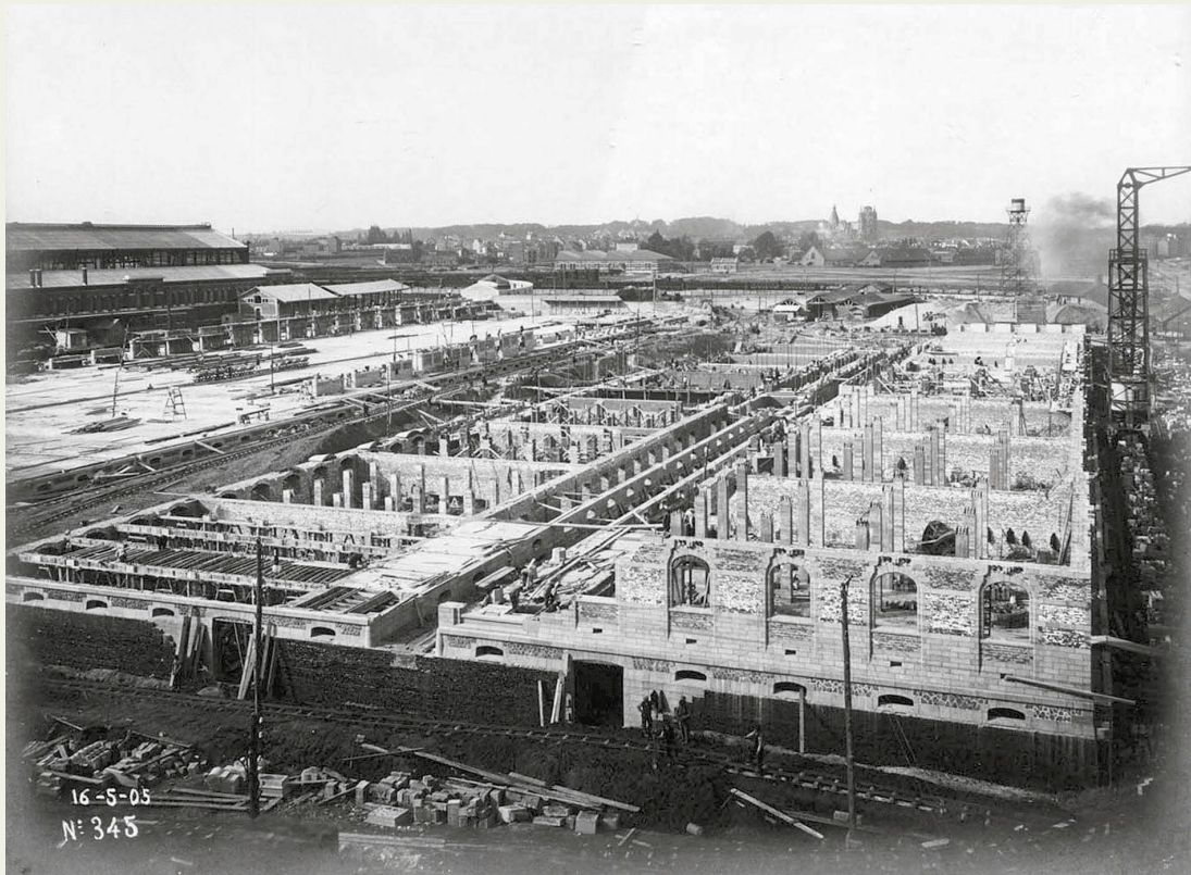
De funderingen van het Koninklijk Pakhuis zijn voltooid, evenals een deel van het metselwerk van de benedenverdieping. Links, langs het goederenstation, is de vloer van het toekomstig entrepot A zichtbaar. In de verte tekent zich het silhouet af van de kerk van Laken.
