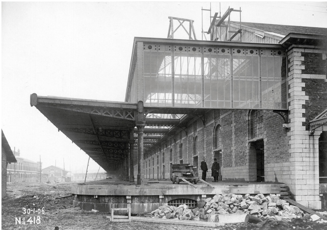
Het brede overdekte perron langs de westelijke gevel van het entrepot met sheddak in 1906. Door de latere verbreding van het gebouw werd het perron afgebroken en een dertigtal meter verder heropgebouwd.
