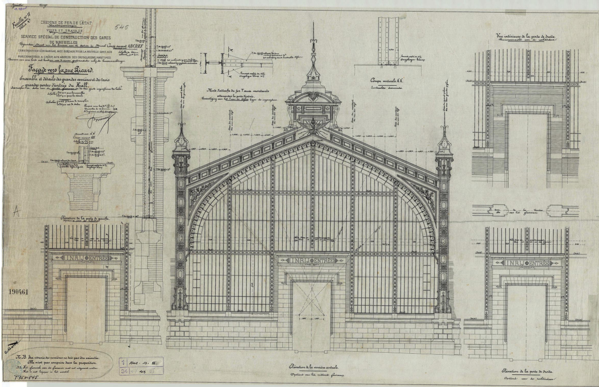
Opstand van de centrale glaswand van het goederenstation dat uitgaat in de Picardstraat. De vele decoratieve elementen in gietijzer en natuursteen van de pinakels en het fronton werden in de jaren 1970 allemaal verwijderd.
