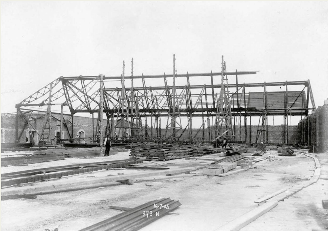
De drie eerste traveeën van het metalen skelet van entrepot A tijdens de montage.
