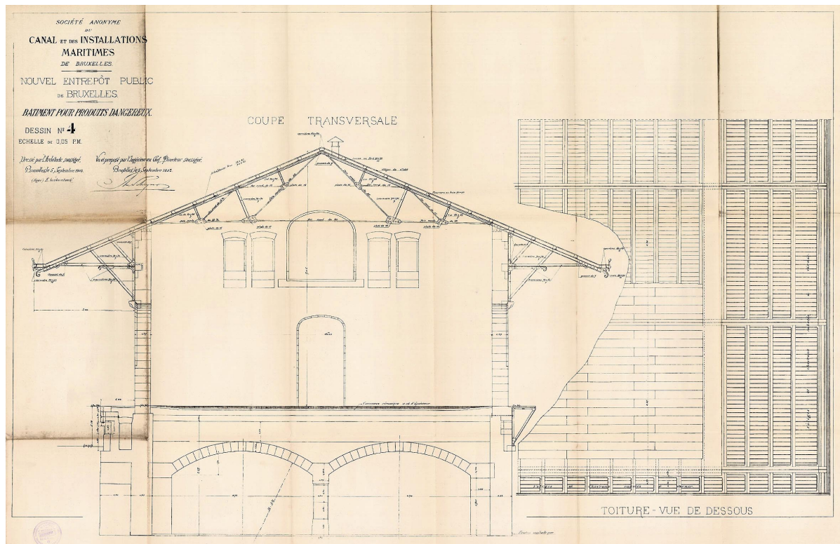
Dwarsdoorsnede die de dunne metalen kapconstructie van het dak laat zien. E. Van Humbeek, 1903.
