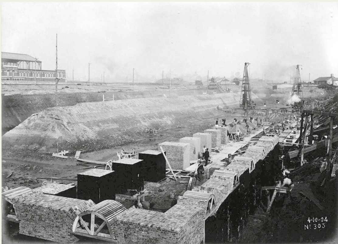
De eerste bakstenen pijlers van het Koninklijk Pakhuis in opbouw terwijl op de achtergrond heismachines funderingspalen in de grond drijven.
