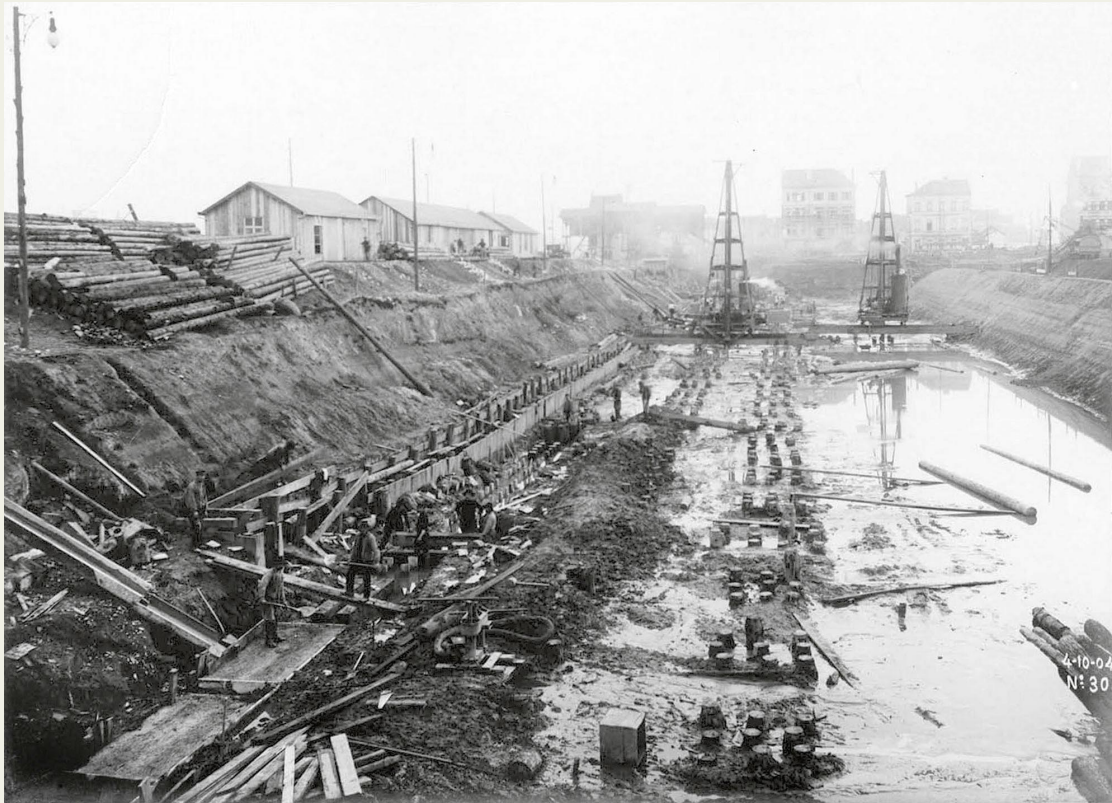
In de uitgraving voor het Koninklijk Pakhuis zijn op de achtergrond twee heimachines bezig met het heien van de funderingspalen.
