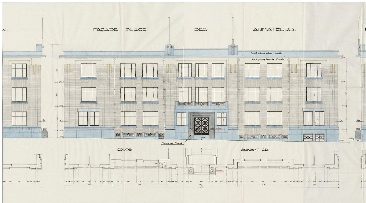
Gevelopstand aan het Redersplein, ontworpen door de hoofdingenieur van de S.A du Canal et des Installations maritimes de Bruxelles , 1938.
