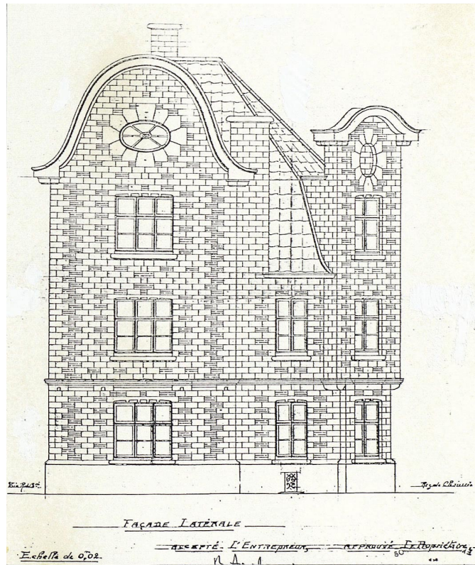
Zijgevel van een van de woningen in de Laekenveldstraat, arch. A. De Saulnier, 1921.
