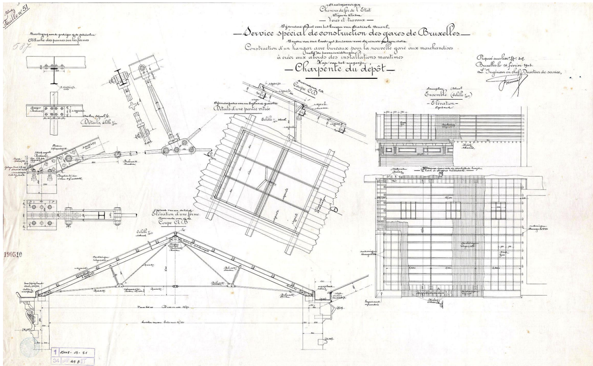
Details van de metalen overkapping van het depot naast het goederenstation.
