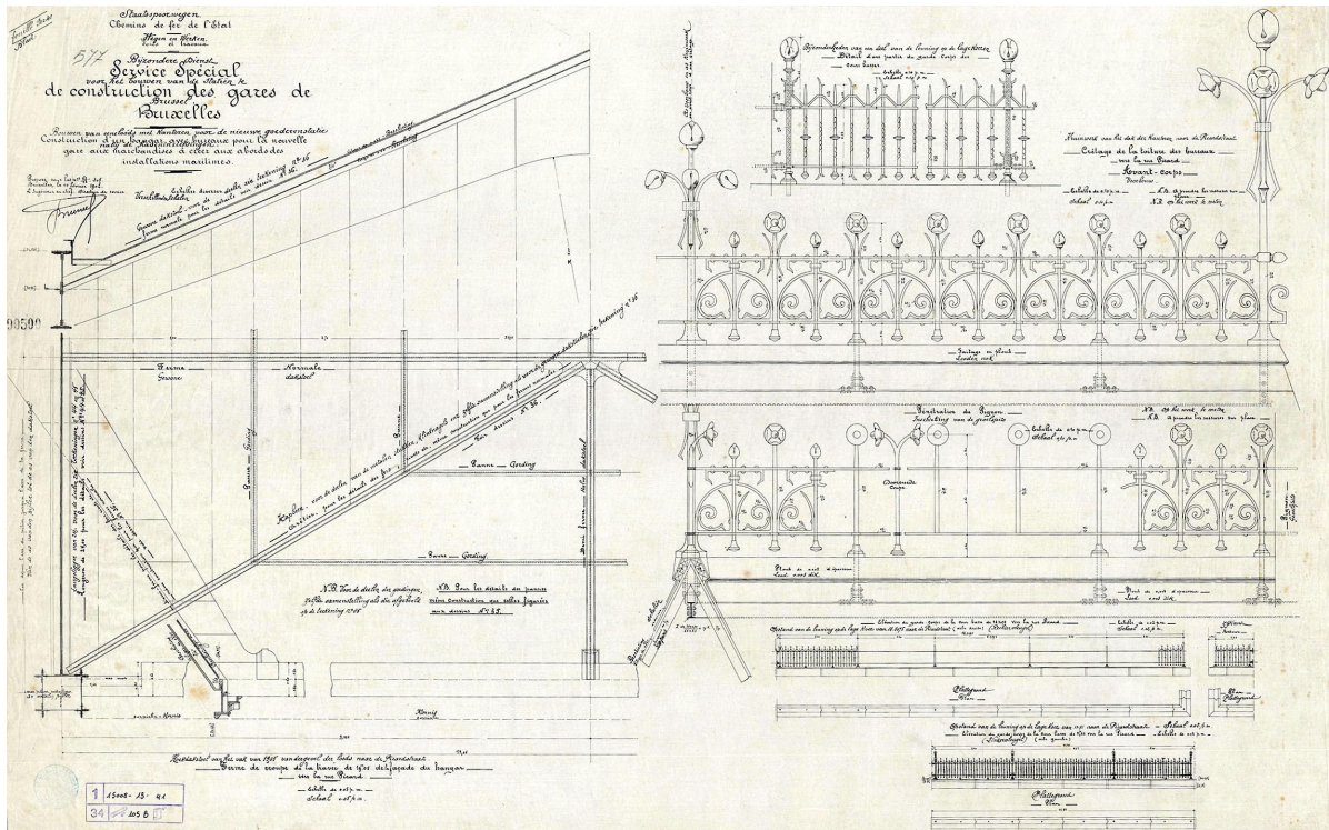
Details van het siersmeedwerk op de nok van het dak – een vandaag verdwenen decorelement – van het administratief gebouw en van de borstwering van de kelderkoeren.
