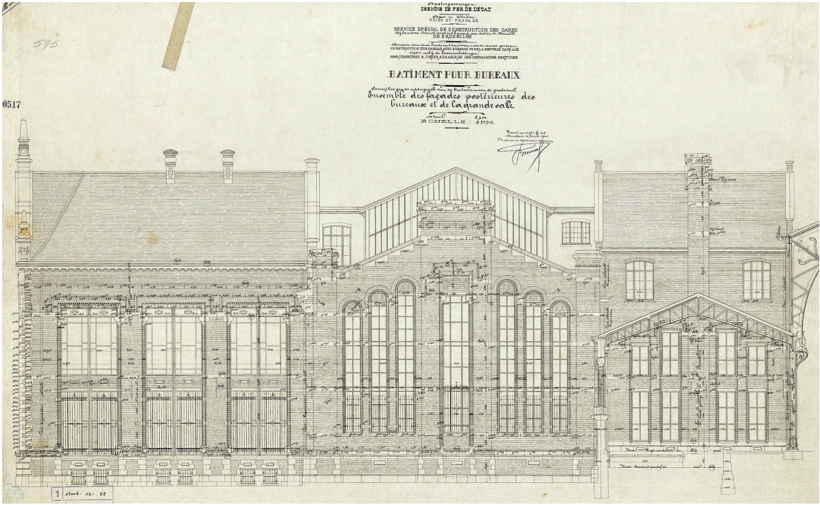
Opstanden van de achtergevel van het administratief gebouw.
