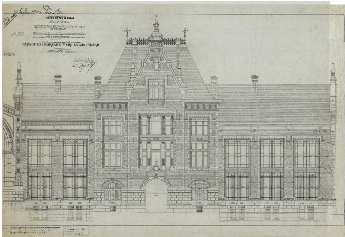
Plannen van 1902: opstand van de gevel van het administratief gebouw dat uitgaat in de Picardstraat.
