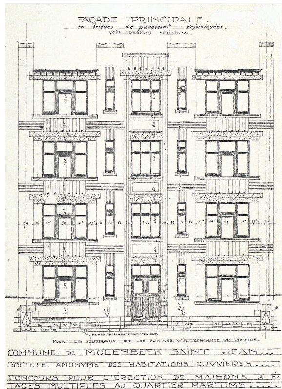
Voorgevel met parement van opgevoegde bakstenen, arch. J. Diongre, 1921.
